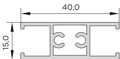
ФСТ-65 Профиль импоста
