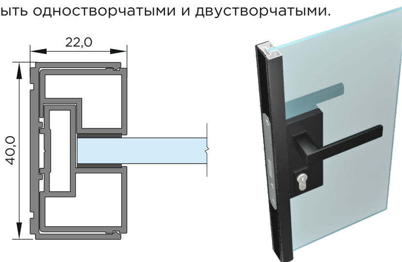
фрагменты сечения дверного полотна Phantom one
