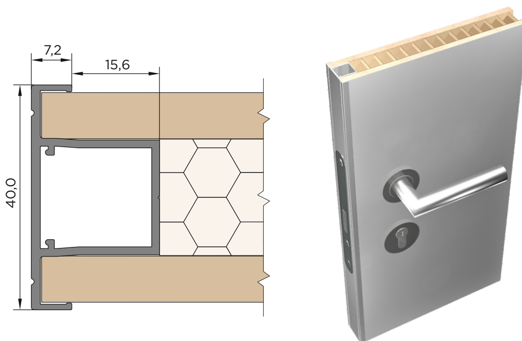
фрагмент сечения дверного полотна Элегант / Elegant
